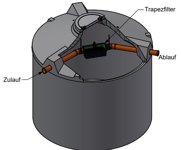
Isometrie
